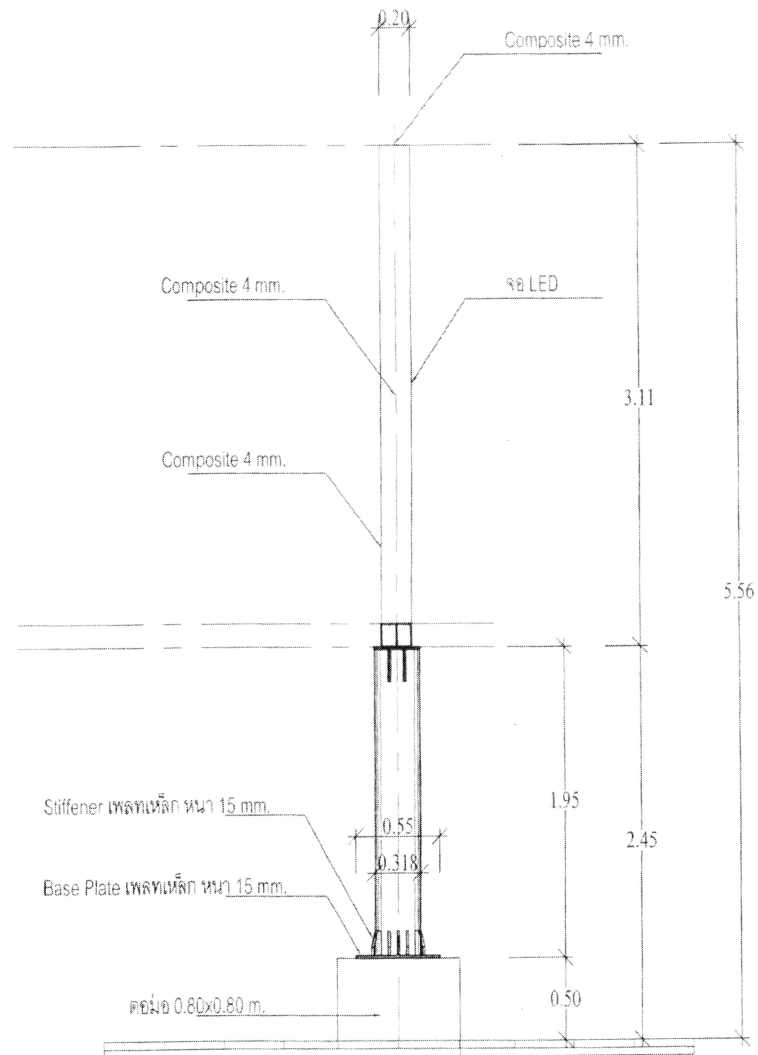
รูปด้านข้าง 1:30
