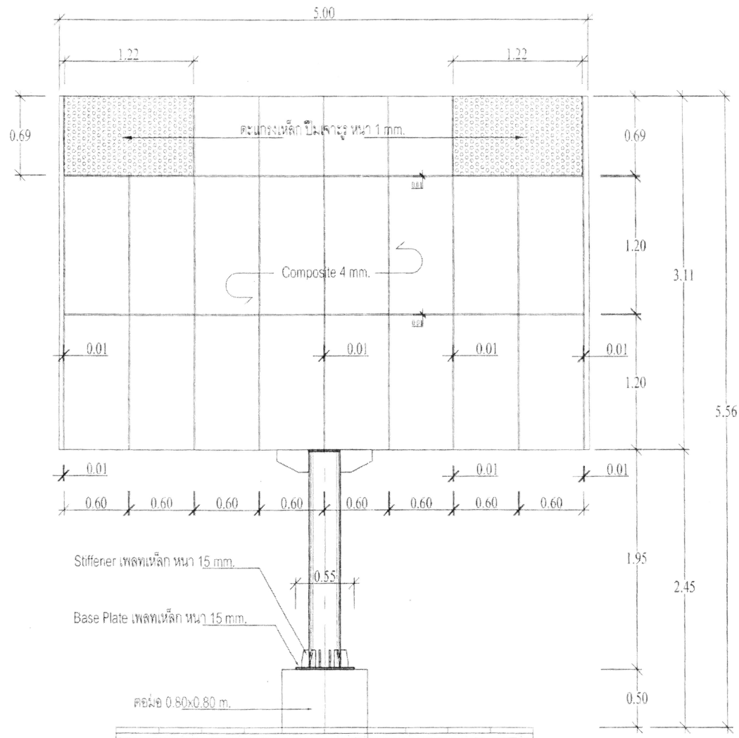
รูปด้านหลัง 1:30
